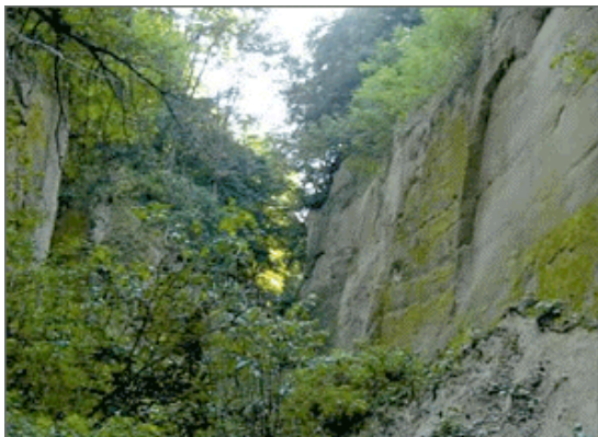
Fig 5: Canionul Mihaileni
